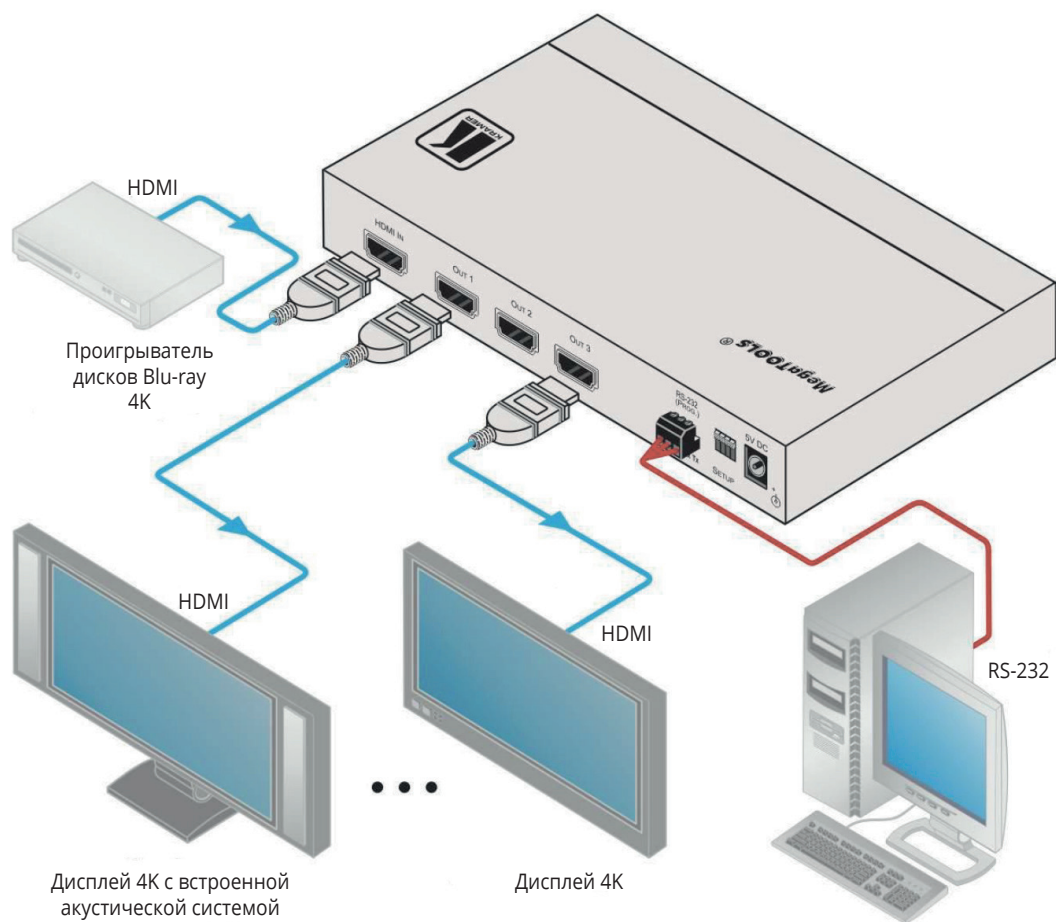
Рис. 2. Подключение VM-3H2
