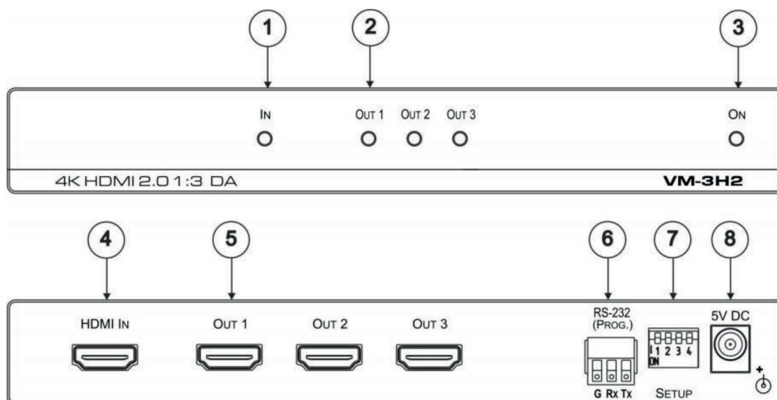
Рис. 1. Вид лицевой и задней панелей VM-3H2
