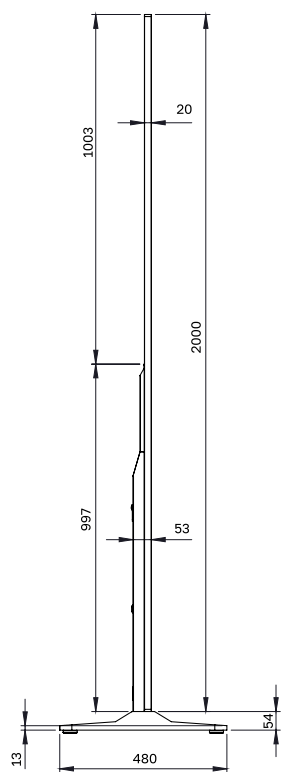
СХЕМА ДИСПЛЕЯ (ВИД СЛЕВА)
