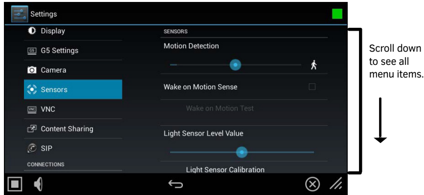
FIG. 38 Sensors page (Available on MDT-2002 model)
