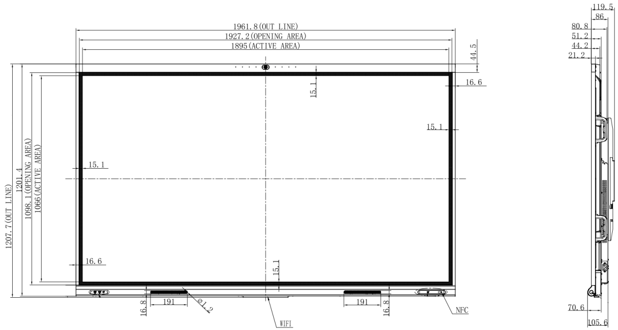
Рис.5 Вид спереди
