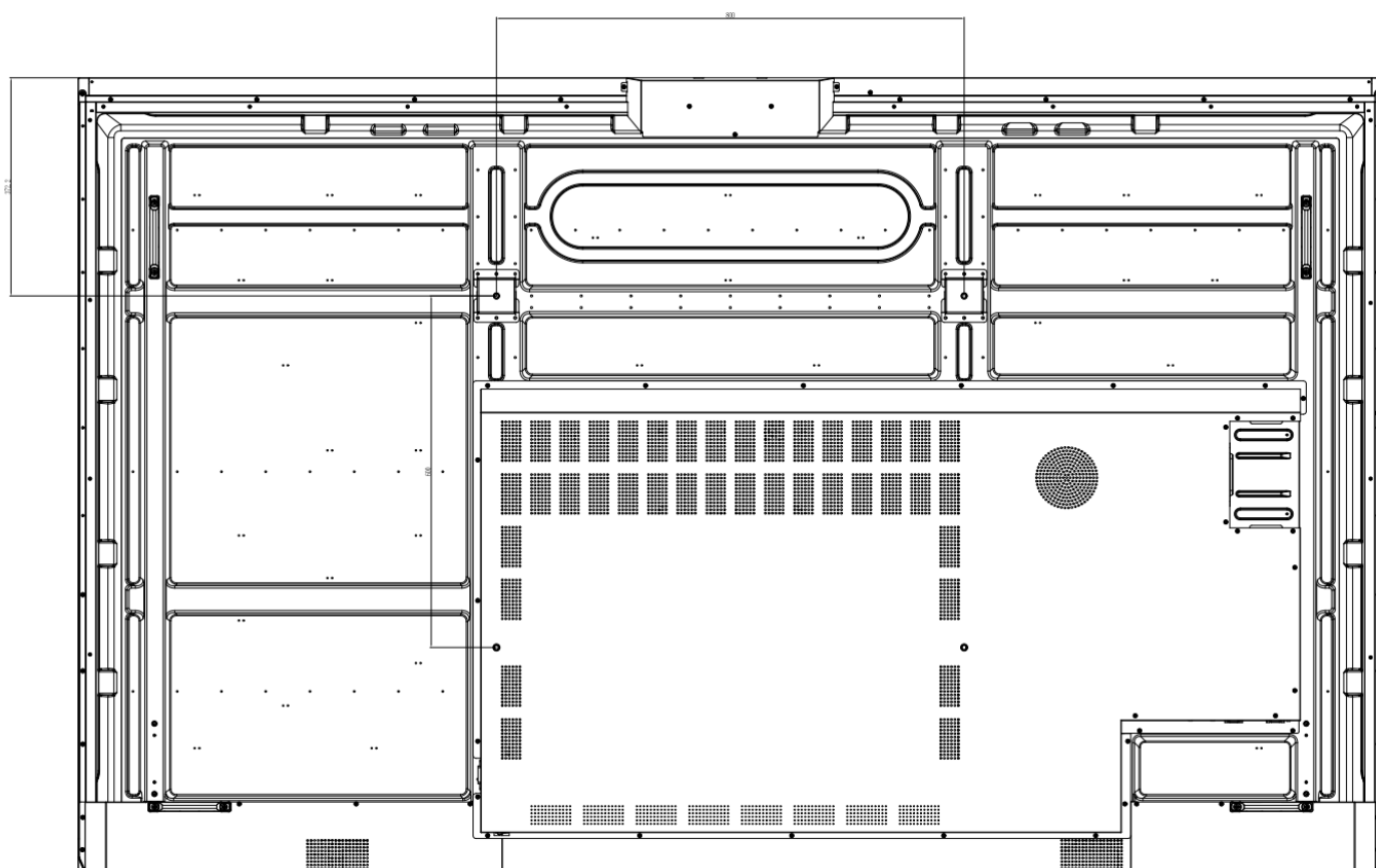
Рис.8 Вид сзади
