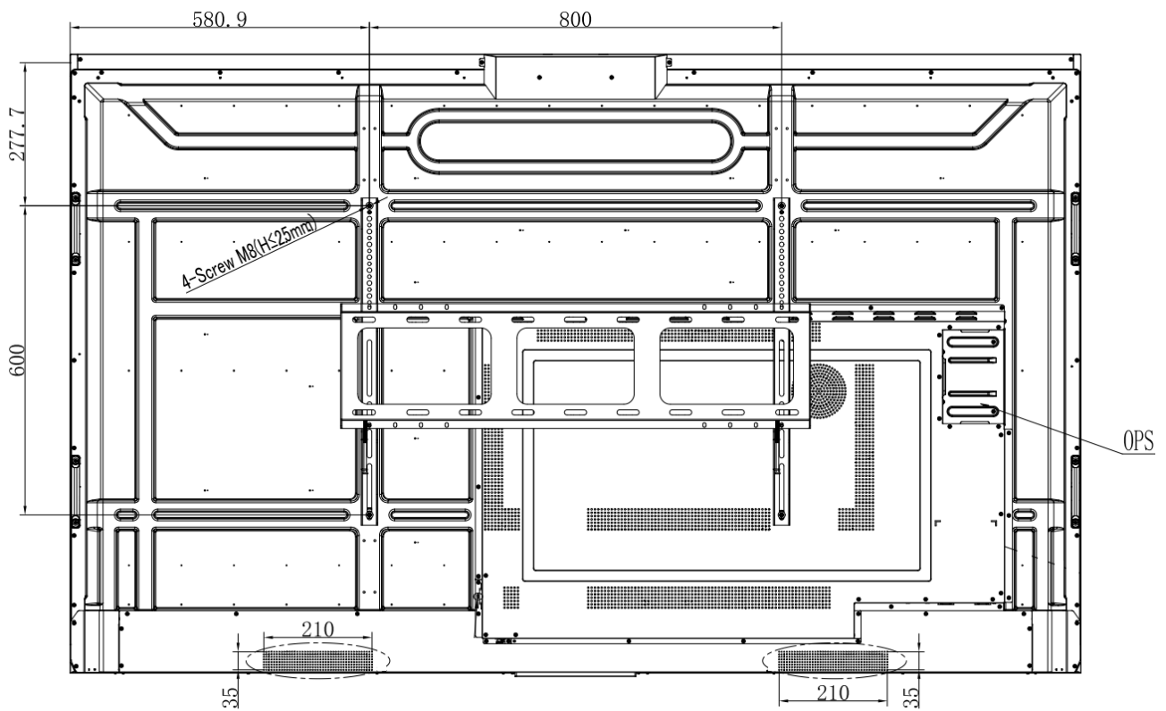
Рис.6 Вид сзади
